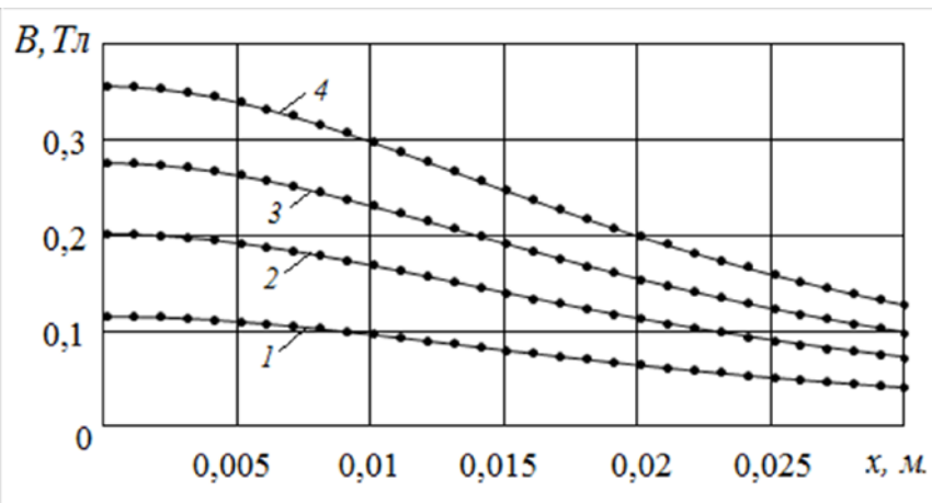
Рис. 6 – Модельные координатные характеристики индукции между полюсами при межполюсном расстоянии 10мм и различных значениях величины тока питания катушек I : 1 – I = 1A ; 2 – I = 2A ; 3 – I = 4A ; 4 – I = 7,5A
