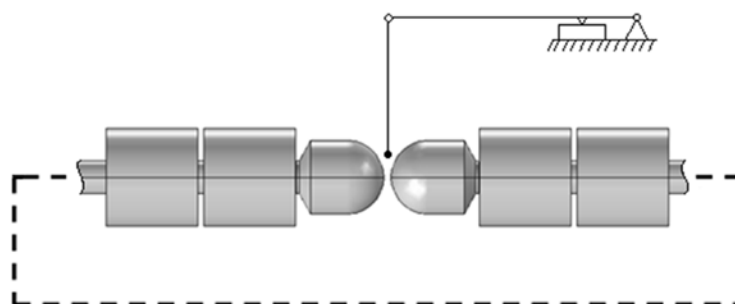
Рис. 4 – Схема магнетометра Фарадея – модернизированного [5], [6], [7]: с применением полюсных наконечников сферической формы
