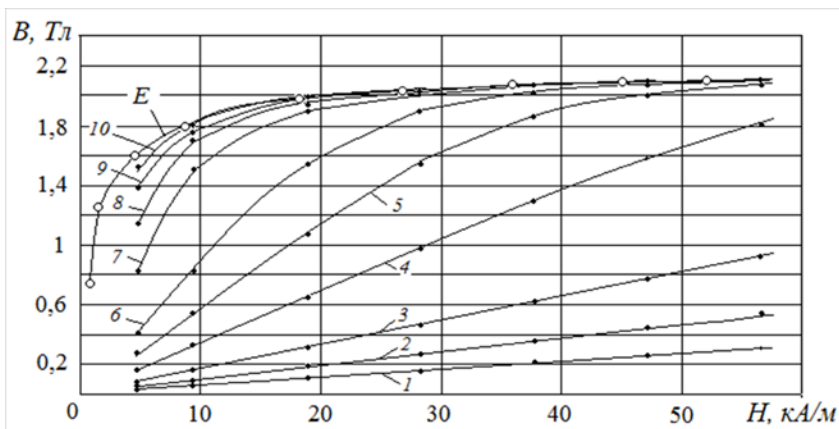
Рис. 2 – Модельные (1-10) полевые зависимости индукции в сплошных «коротких» образцах – с различными значениями L/D : 1 – L/D = 1 ; 2 – L/D = 1,8 ; 3 – L/D = 3 ; 4 – L/D = 5,5 ; 5 – L/D = 8 ; 6 – L/D = 11 ; 7 – L/D = 19 ; 8 – L/D = 25 ; 9 – L/D = 32 ; 10 – L/D = 43 ; кривая E – экспериментальная зависимость для сплошного, достаточно «длинного», образца: L/D = 50
