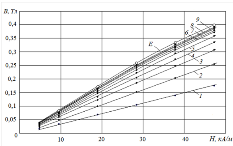
Рис. 3 – Модельные (1-9) полевые зависимости индукции в гранулированных «коротких» образцах – с различными значениями L/D : 1 – L/D = 1,01 ; 2 – L/D = 2,04 ; 3 – L/D = 3,12 ; 4 – L/D = 4,11 ; 5 – L/D = 5,43 ; 6 – L/D = 6,78 ; 7 – L/D = 8,27 ; 8 – L/D = 9,4 ; 9 – L/D = 12,9 ; кривая E – экспериментальная зависимость для гранулированного (засыпка шаров), достаточно длинного, образца: L/D = 16
