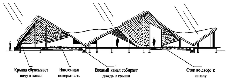
Рисунок 5 - Вид в разрезе роли крыши и системы каналов для приема и отвода дождевой воды
