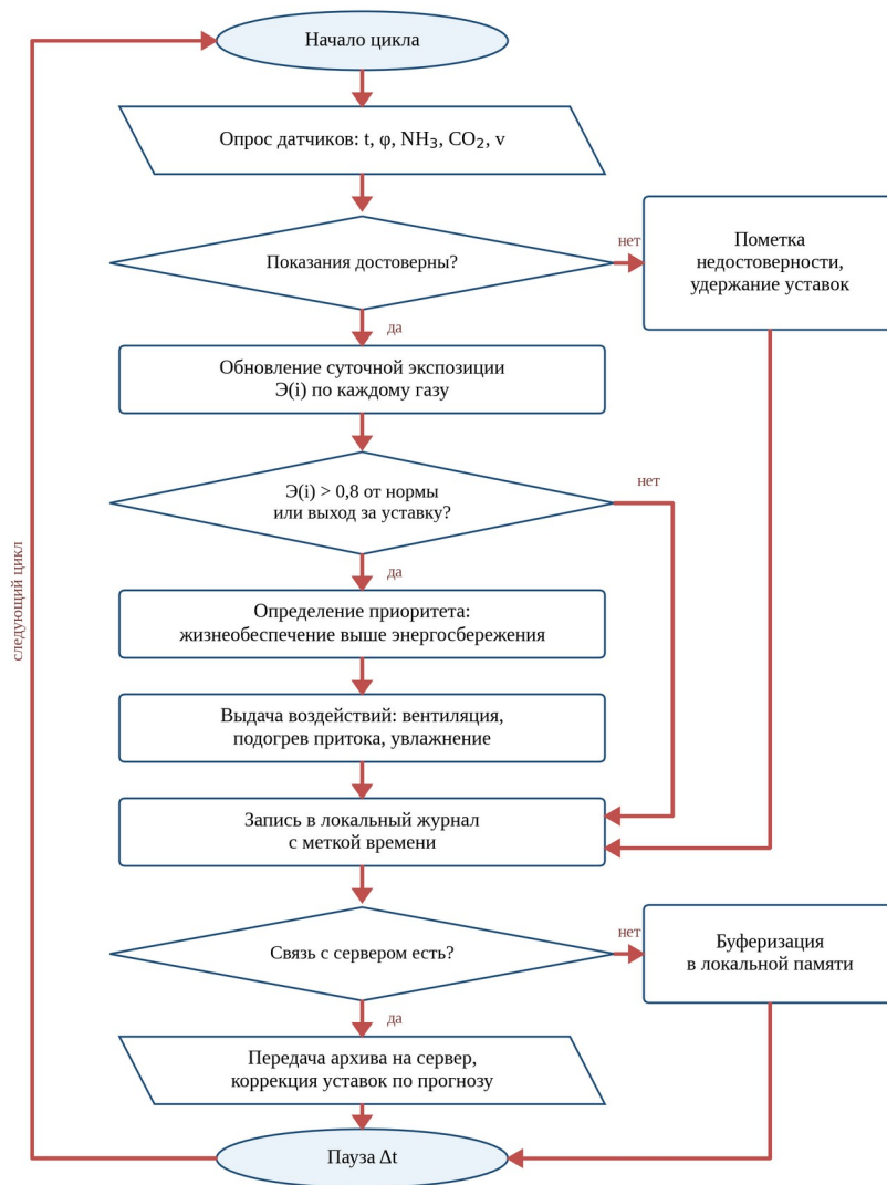
Рисунок 2 - Схема алгоритма работы системы DOI: https://doi.org/10.60797/IRJ.2026.172.34.2
