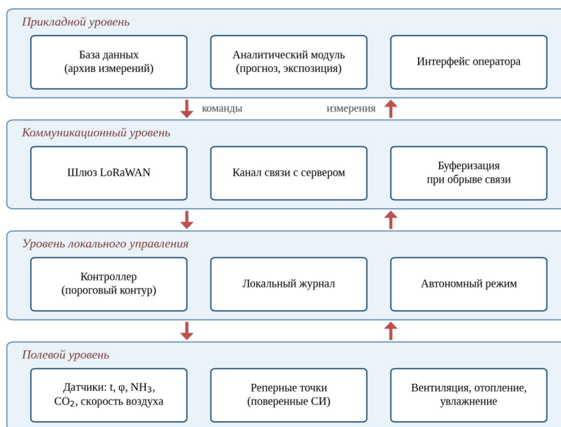
Рисунок 1 - Структура системы удалённого мониторинга и управления микроклиматом животноводческого помещения
