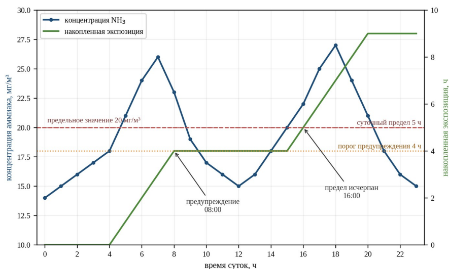
Рисунок 3 - Суточный ход концентрации аммиака и накопленная экспозиция DOI: https://doi.org/10.60797/IRJ.2026.172.34.3
