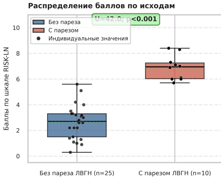
Рисунок 5 - Распределение баллов шкалы RISK-LN DOI: https://doi.org/10.60797/IRJ.2026.167.24.5
