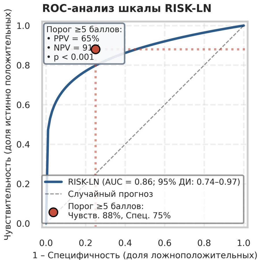
Рисунок 4 - ROC кривая
